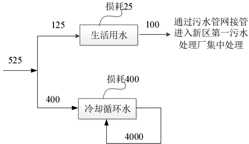
图 5-2 本项目水平衡图 (t/a)
